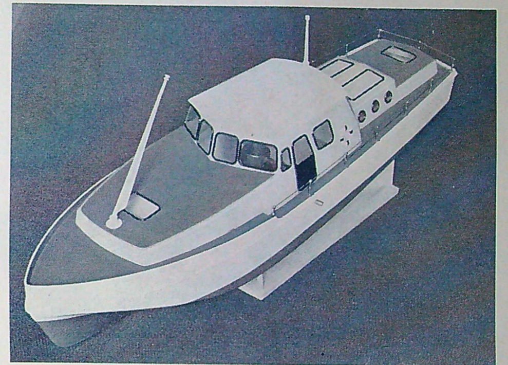
Monte Carlo färdigbyggd. Byggsatsen har alla delar färdiga för montering och utom plastdelarna medföljer propelleraxel med lagertrumma och propeller — för elmotor — samt lim.
