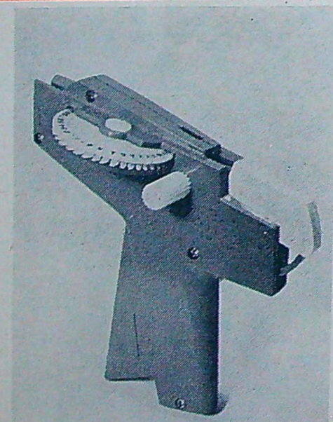
På bilden syns de båda avtryckarna tydligt. Genom att trycka in den stora avtryckaren endast till strecket matas bandet fram ett steg utan präglning (mellanlag).
