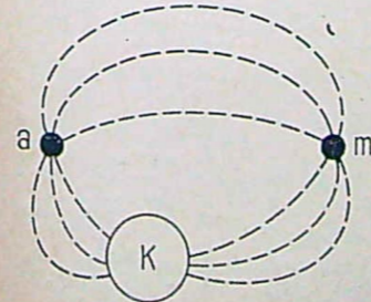
Mellan elektroden a och m spänner ett elektriskt fält (streckade linjer). Kommer en kropp (K) in i fältet så förändras fältstyrkan och därmed utlöses larmet.
