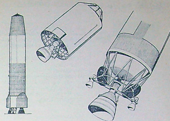
Satellitbäraren ELDO-A (Europa 1): I v Steg 1: Blue Streak. I mitten Steg 2, det franska Coralie, i h det västtyska Steg 3, från ERNO.
