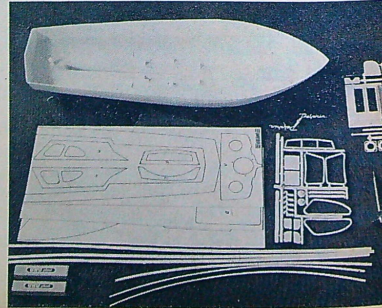
Detta är byggsatsen till Delphin. Fortuna-satsen har ett liknande utseende. Skrovet har en längd av 69 cm och en största bredd på 20 cm.
