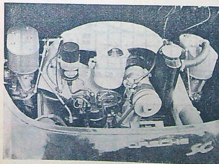
På CS-modellen har motorstyrkan ökat från 90 till 95 hk, vilket främst kommit accelerationen till godo. Det ser trångt ut i motorrummet, men sådant som ofta måste justeras är lätt åtkomligt.
