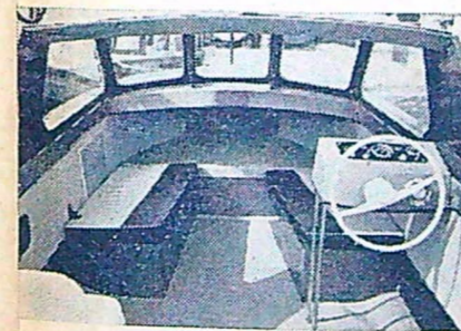
Kabinen saknar akterskott, dvs den är öppen akterut. Styrplatsen är därför arrangerad som en manöverpulpet.
