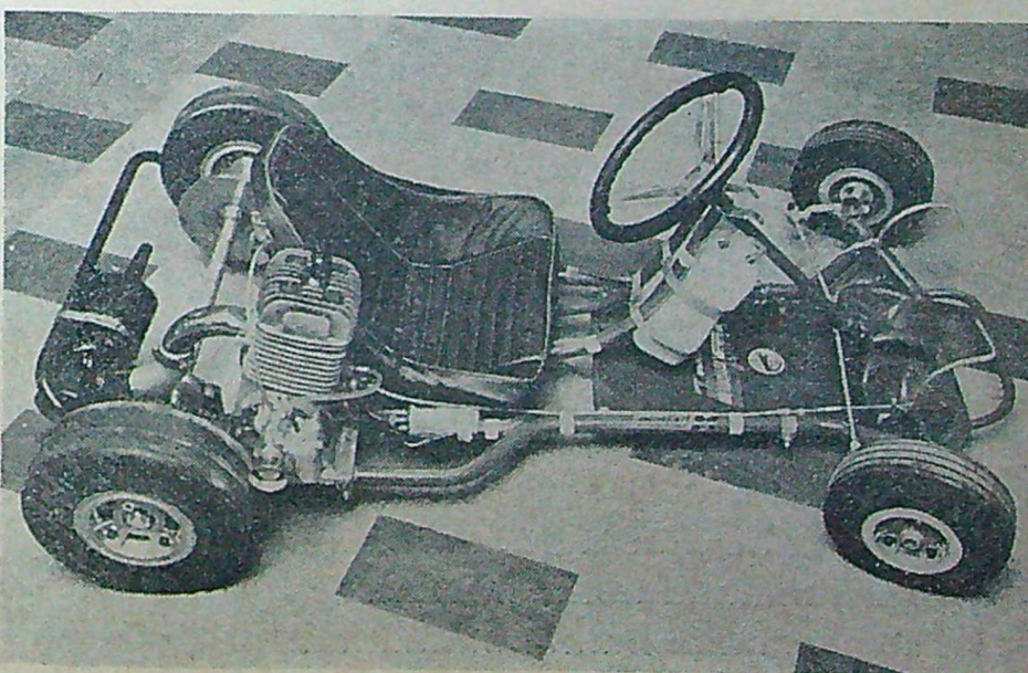
Denna placering av motorn godkänns. Men var finns skiljeväggen för brandskyddet mellan föraren och motorn?
