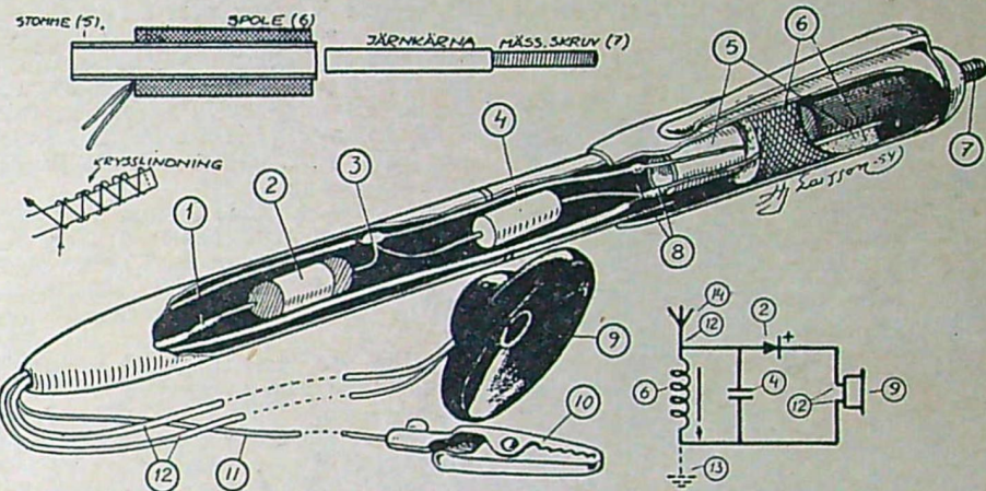
1) Den ena sladden till hörluren löds fast vid plusuttaget på kristalldioden. 2) Kristalldiod. 3) Kristalldiodens andra uttag löds här fast vid antennen. Likaså kondensatorns ena uttag. 4) Kondensator. 5) Spolstomme. 6) Lindning med litztråd. 7) Mässingskruv med vilken järnkärnan kan skruvas in eller ur spolen. 8) Spolens ena ände löds fast vid antennen och den andra vid kondensatorns andra ände och hörlurens andra sladd. Se till att trådarna är väl isolerade innan det hela monteras in i pennan. 9) Hörlur. 10) Liten krokodilklämma. 11) Antennsladd. 12) Sladdar till hörlur. 13) Jordledning, om så önskas. Den löds i så fall fast vid spolens nedre tråd vid 8 och dras ut i pennans ände. 14) Antenn, som kan bestå av vilket metallföremål som helst.
