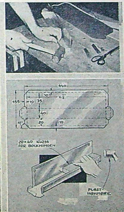
Fig. 8 (t. v.): På insidan av en skåpdörr kan hyllor av aluminium sättas upp, såsom visas längst t. v. De båda övriga bilderna visar hur tillverkningen tillgår. Fig. 9 (bilderna ovan): Överst ett toalettstap i vilket finns en extra hylla av aluminium. Teckningen ovan visar hyllans konstruktion och av bilden i mitten framgår hur den förädlas.
