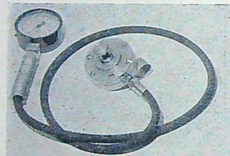
Pressometern möjliggör effektiv bromskontroll.
