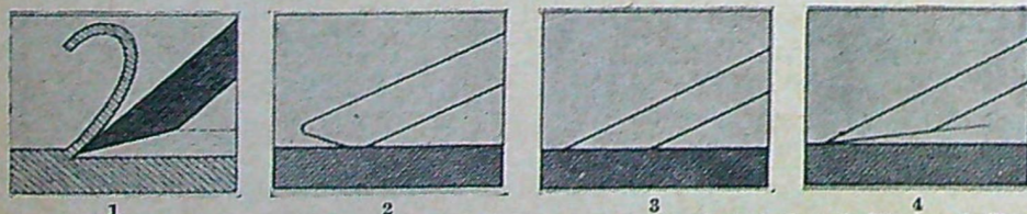
Fig. 2: 1. visar hur ett korrekt hyvelstål ligger an mot arbetsstycket. 2. Ett hyvelstål som behöver justeras, dels är bladvinkeln för trubbig och dels behöver eggen skärpas. 3. Visar hur stålet ska ligga an mot brynet under skärningen. 4. Visar hur eggvinkeln silpas in under finskärpning.
