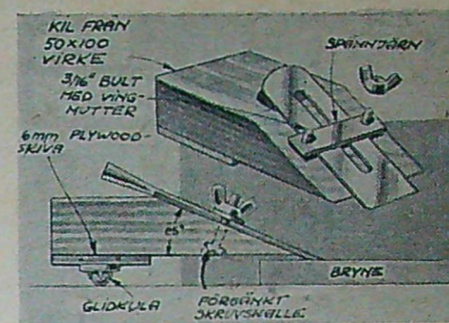
Fig. 3 (ovan): En Jigge för skärpning av hyvelstål och stämjärn kan tillverkas med ledning av figuren.
