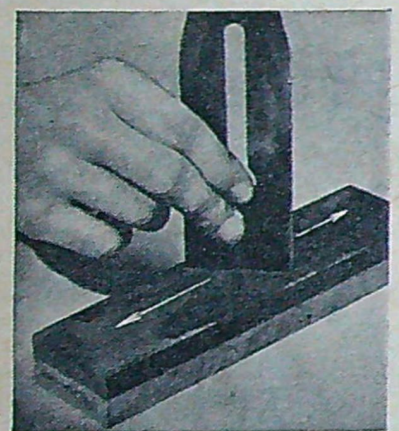
Sedan justeras eggen i rät linje om så erfordras. Detta görs genom att stålet dras mot brynet i vertikalt läge. Kontrollera med en vinkelhake att eggen blir rak och i rät vinkel med stålets sidkanter.
