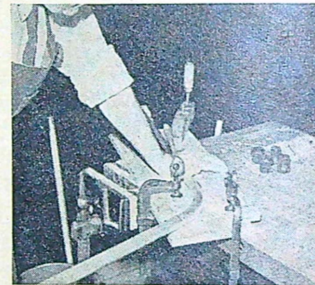
Fig. 5. Aluminiumrören till bordet bockas runt en mall sedan de packas med våt sand vilket gör att de inte plattas till i kröken.
