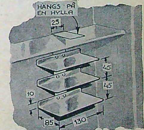
Fig. 8 (t. v.): På insidan av en skåpdörr kan hyllor av aluminium sättas upp, såsom visas längst t. v. De båda övriga bilderna visar hur tillverkningen tillgår. Fig. 9 (bilderna ovan): Överst ett toalettstap i vilket finns en extra hylla av aluminium. Teckningen ovan visar hyllans konstruktion och av bilden i mitten framgår hur den förädlas.
