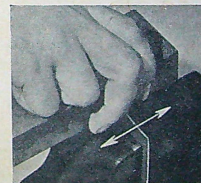
För skärpning av ett skrapstål bör stålet sättas fast i ett skruvståd. Först silpas stålet med ett grovt bryne och slutligen med ett fint.
