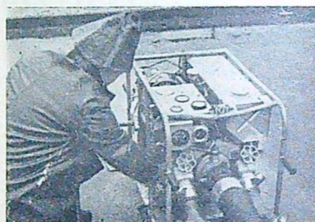
Bilden visar den engelska brandpump som bygger på den lilla gasturbin för stationärt bruk på 60 hk som konstruerats av Rover. Denna gasturbin kombinerad med en snabb centrifugalpump har skapat ett lätt men effektivt pumpaggregat med en kapacitet av 2275 l/m.
