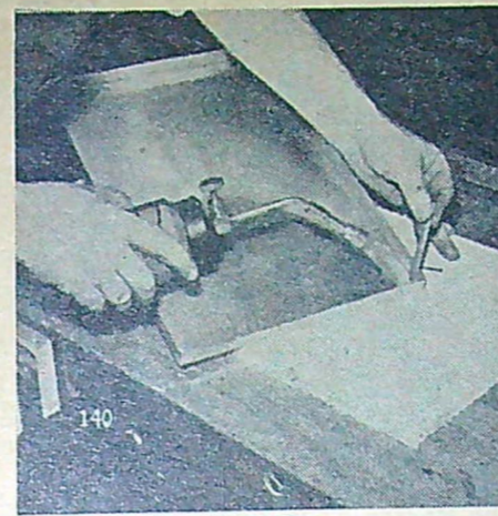
Fig. 7 (bilderna t. v. och t. h.): Gräddplåtar av aluminium är mycket bekväma. Hörnen löds samman med aluminiumlod. Med vanligt lödtenn går lödningen inte att utföra.
