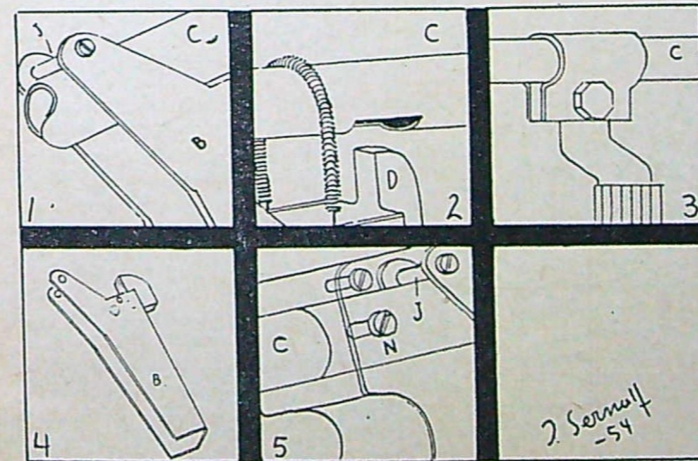
Detaljskisser som visar harpungevärets konstruktion.
