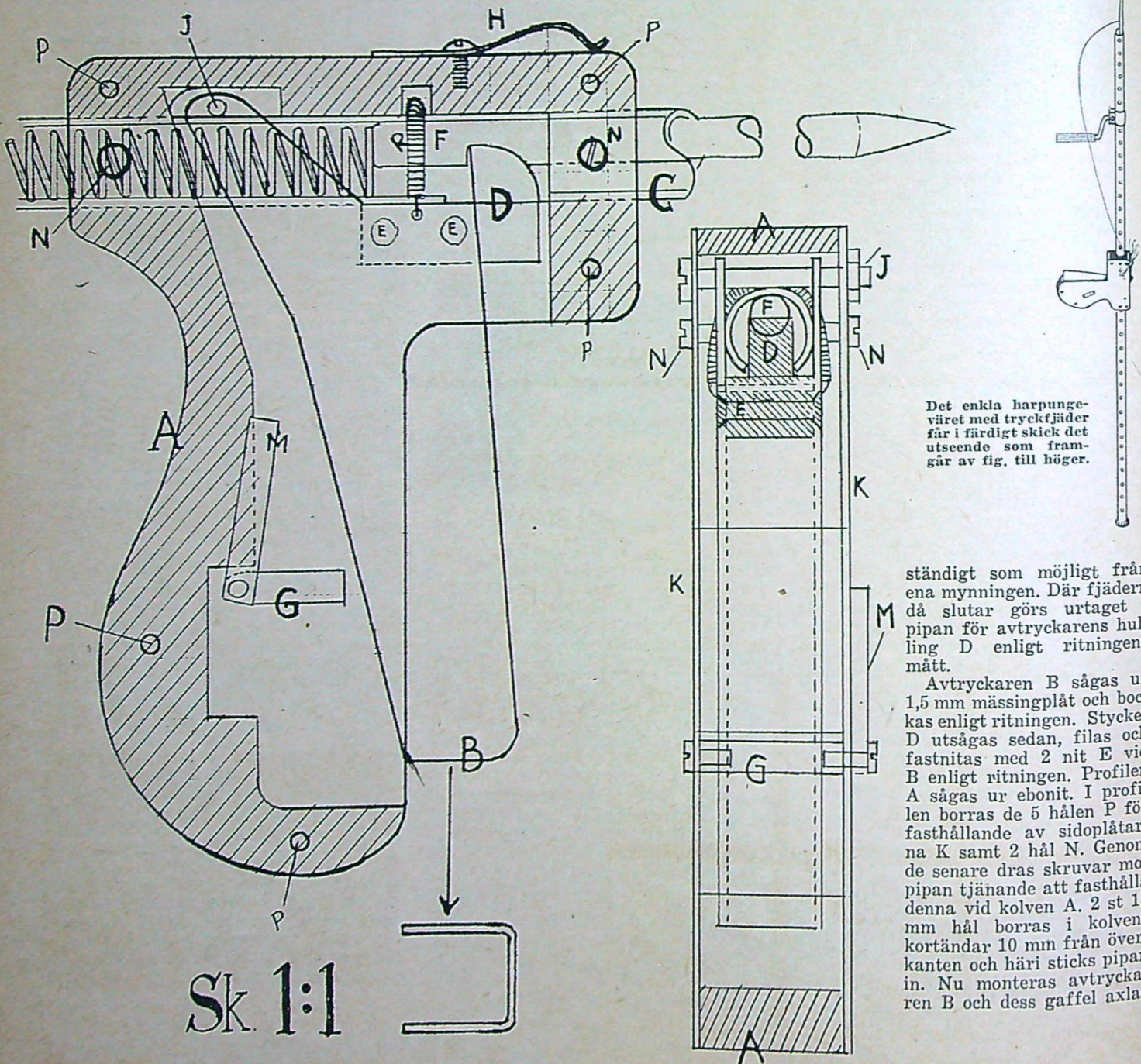
Hur harpungevärets mekanism tillverkas framgår av ritningen nedan. Kolven görs av ebonit (t. h.). Bokstavshänvisningar i texten.
