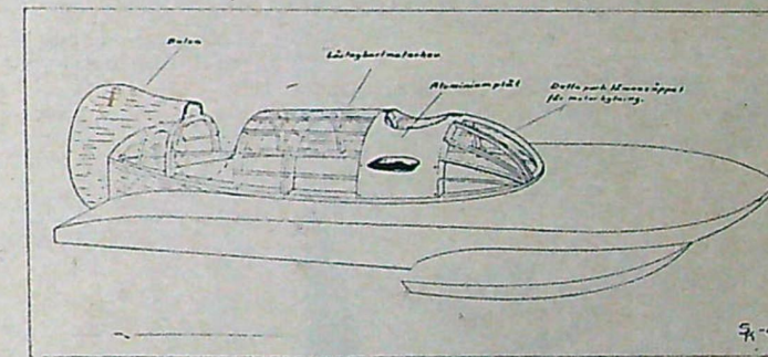
Byggnadsritningar över däcksöverbyggnaden och längst ner t. h. detaljskiss över propellermekanismen.
