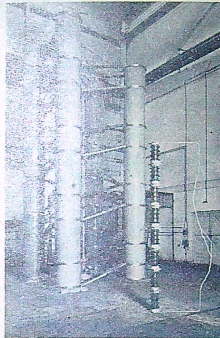
Bilden visar när 2½ miljoner volt hoppar över i ett gnistgap, på ca 2,5 meter.
