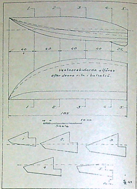
Detaljritning över ventnorskidorna.
