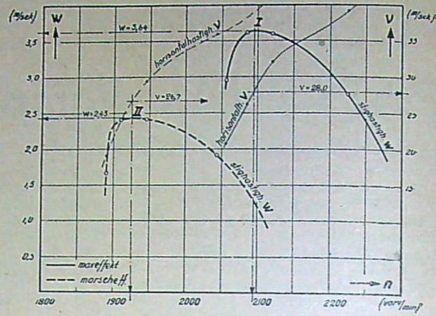
Fig. 20. Med maxeffekt är stighastigheten w 3,64 m/sek vid 2 090 r/m och med marscheffekt 2,43 m/sek vid 1 925 r/m.
