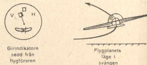
Bild 5. Exempel å instrumentutslag i vänstersväng.
