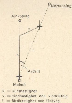
Bild 2. Exempel å vindtriangel och färdväg.
